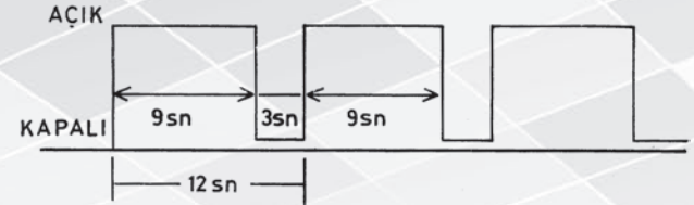
Şekil 12: Zaman oransal kontrol
