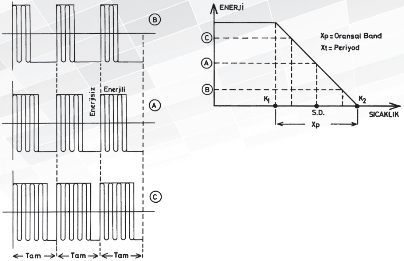
Şekil 14: Zaman oransal kontrol formu
