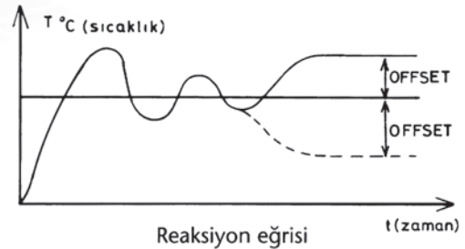
Şekil 6: Geniş oransal band ve reaksiyon eğrisi.
