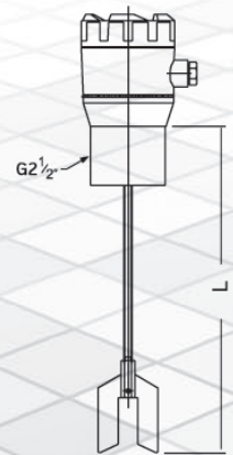
Çift Kanatlı Pervane
