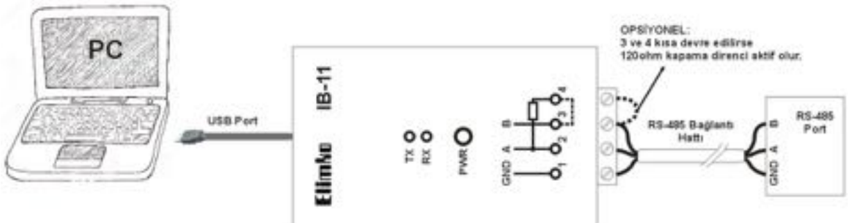
Şekil-3 IB-11 Bağlantı Diyagramı
